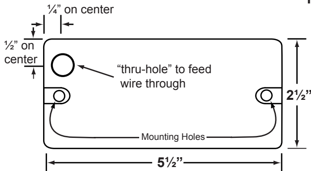
CL-345B-AB SHOWN
